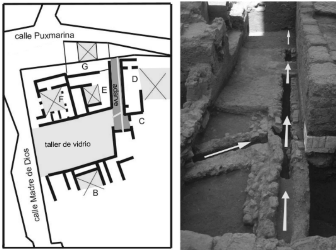
Figura 21. Adarve hallado en las excavaciones arqueológicas del casón de Puxmarina (Murcia). Apréciase la posición descentrada de la atarjea, como resultado de la invasión parcial de la calle por parte de la casa D. La línea original vendría determinada por la alineación de la fachada C y, por tanto, en origen la atarjea corría, como es normal, por el centro del callejón.
