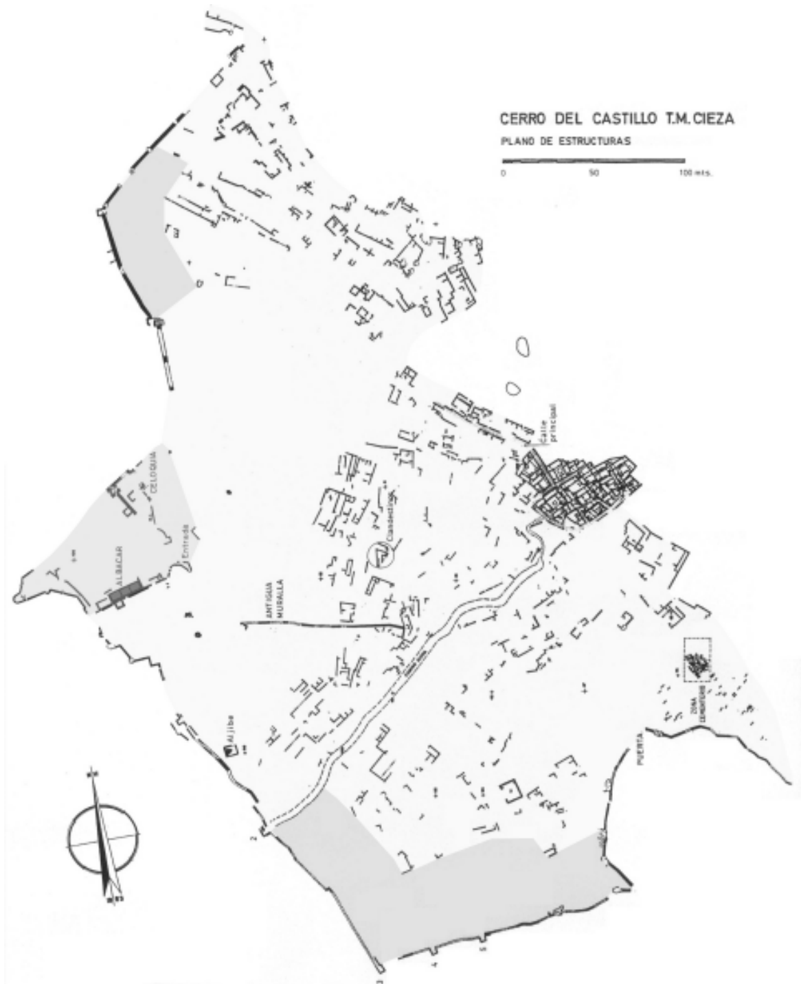
Figura 2. Despoblado de Siyasa (SS. XII-XIII). Planta del yacimiento con los restos visibles y situación del área excavada, la alcazaba y el cementerio. Se han destacado los sectores periféricos, entre el caserío y la muralla, que nunca llegaron a ser urbanizados.
