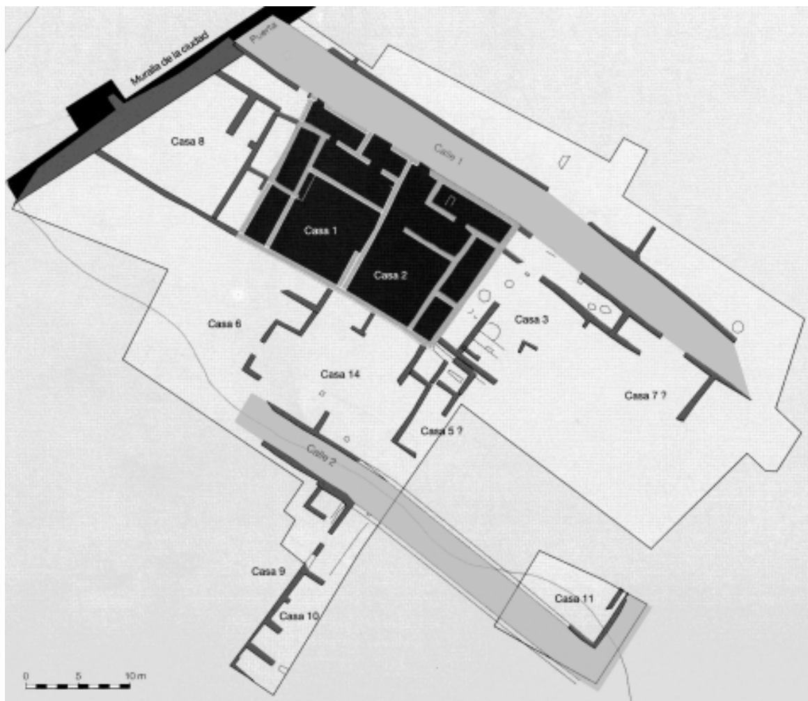
Figura 19. Manzana de casas en el Llano de Almatá, Lérida (s. XI). Se han destacado las dos casas producto de la partición de una gran vivienda original.
