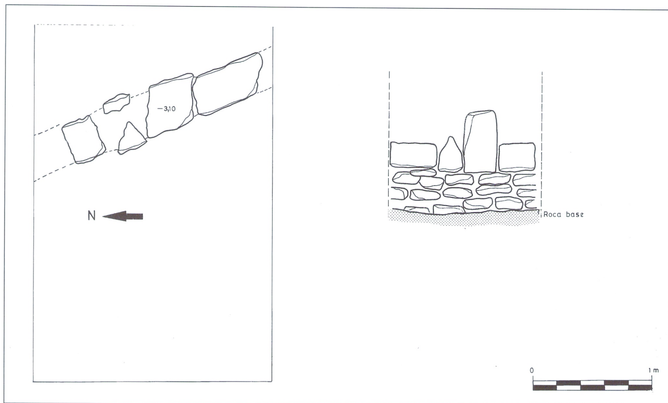
Figura 2. Corte A2. Planta y alzado del muro.
