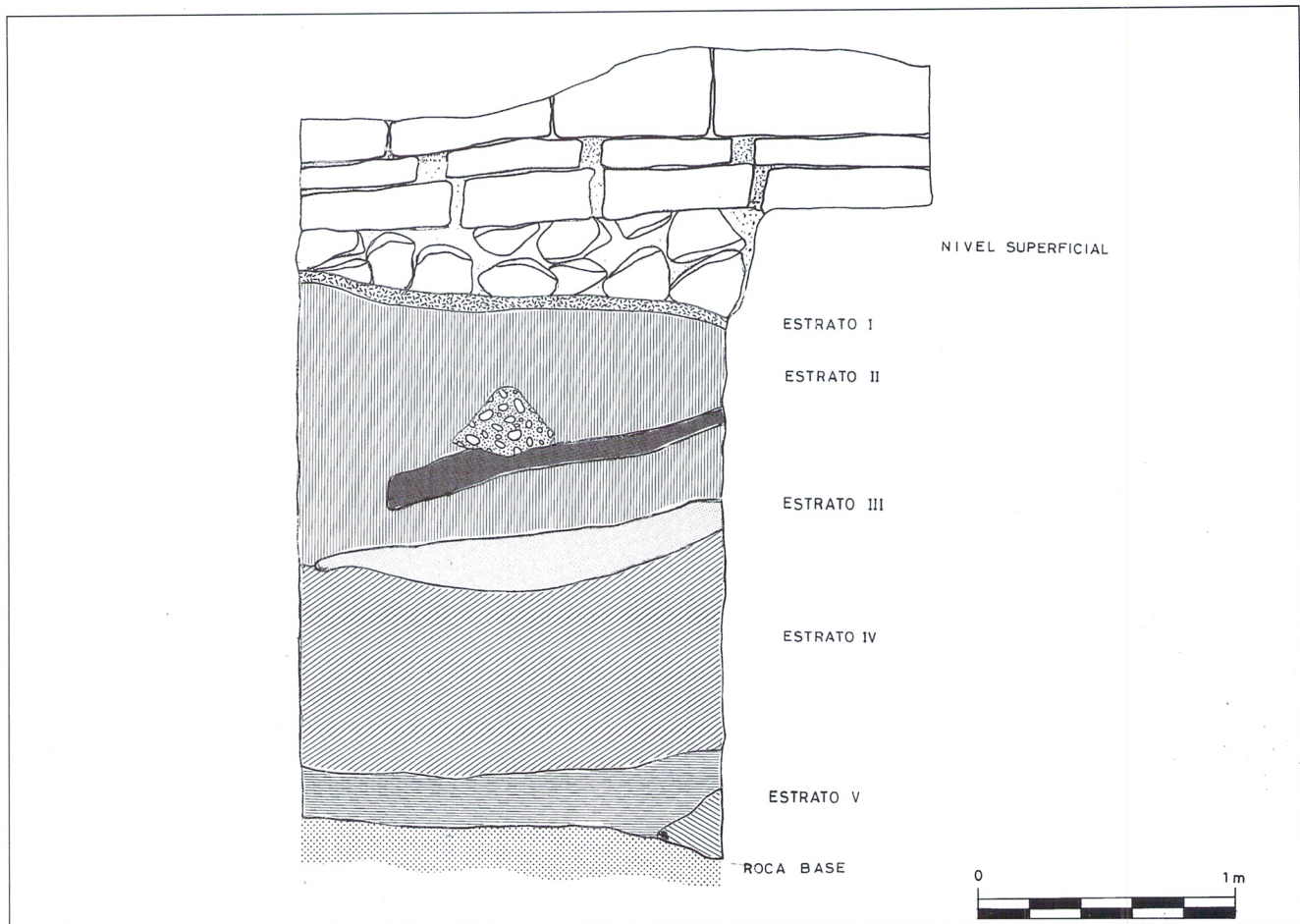
Figura 3. Corte A1. Perfil Norte.
